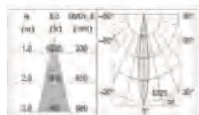
15°-3000K-CRI90
