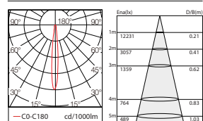
15°-3000K-CRI90
