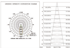
36°-3000K-CRI90
