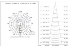
15°-3000K-CRI90
