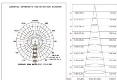
24°-3000K-CRI90
