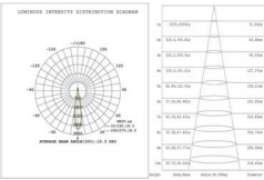
15°-3000K-CRI90
